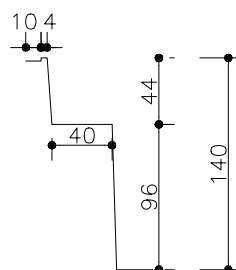
BB CORTE BB ESCALA 1:50
