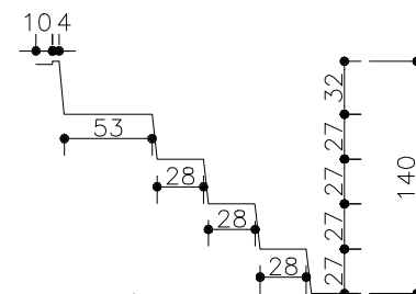
CC CORTE CC ESCALA 1:50
